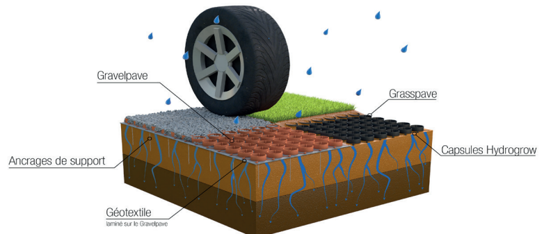
GRASSPAVE2 / GRAVELPAVE2
